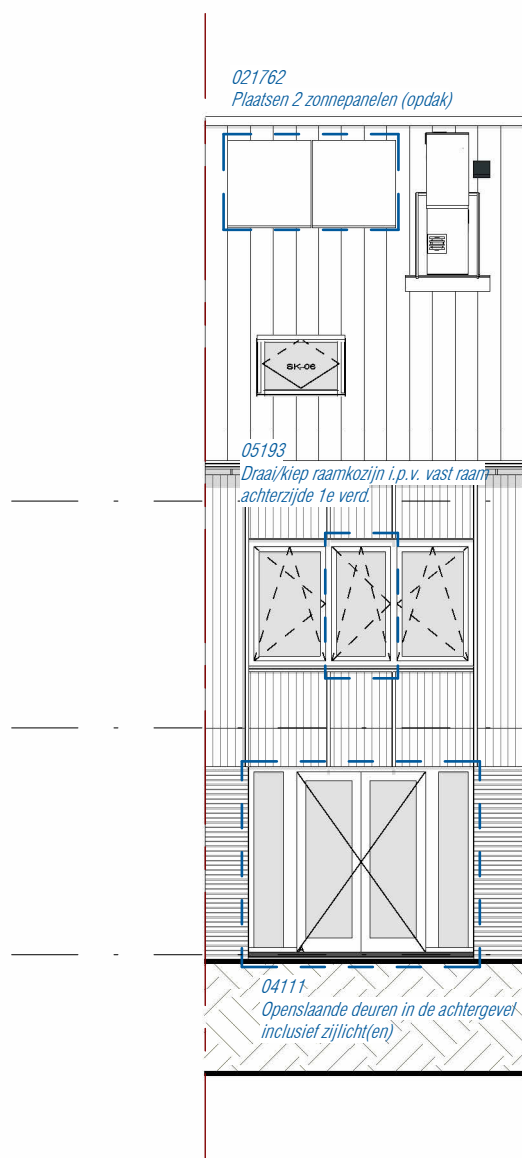
achtergevel 1 : 100
