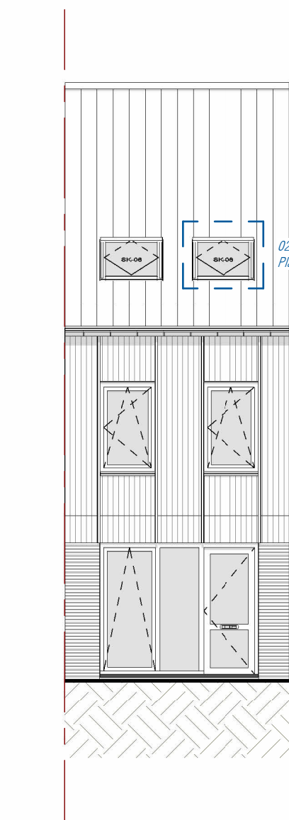
voorgevel 1 : 100
