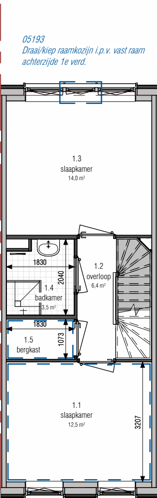
1e verdieping 1 : 100
