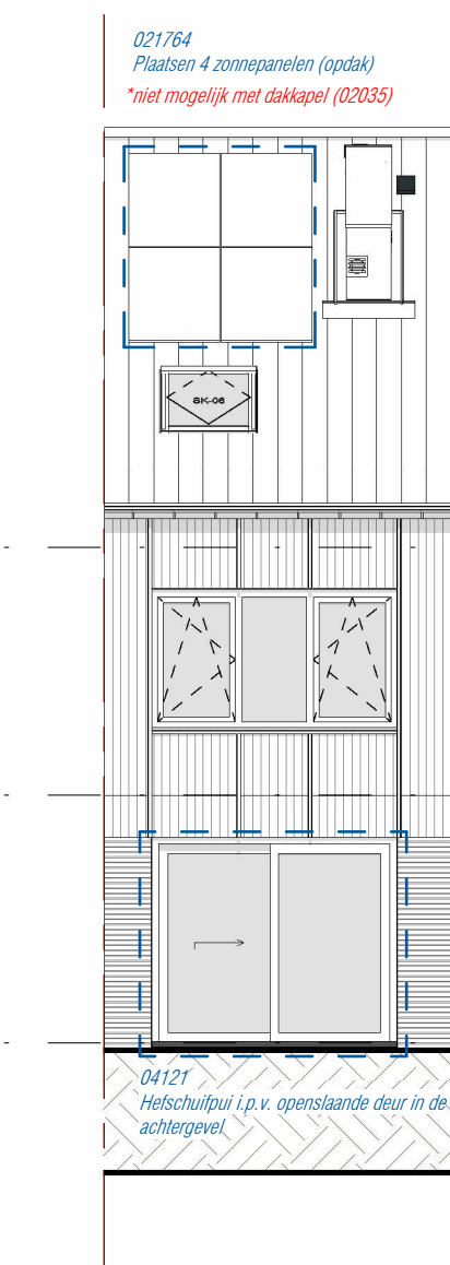
achtergevel 1 : 100
