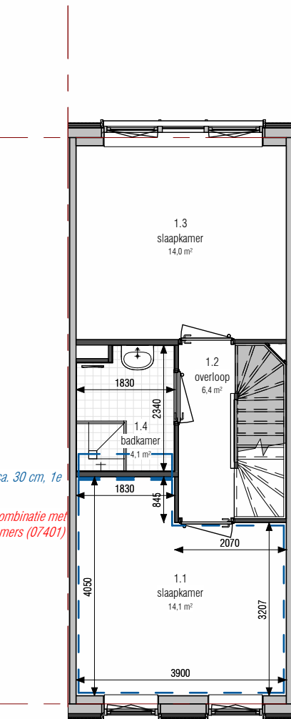
1e verdieping 1 : 100
