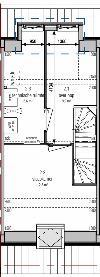
2e verdieping 1 : 100
