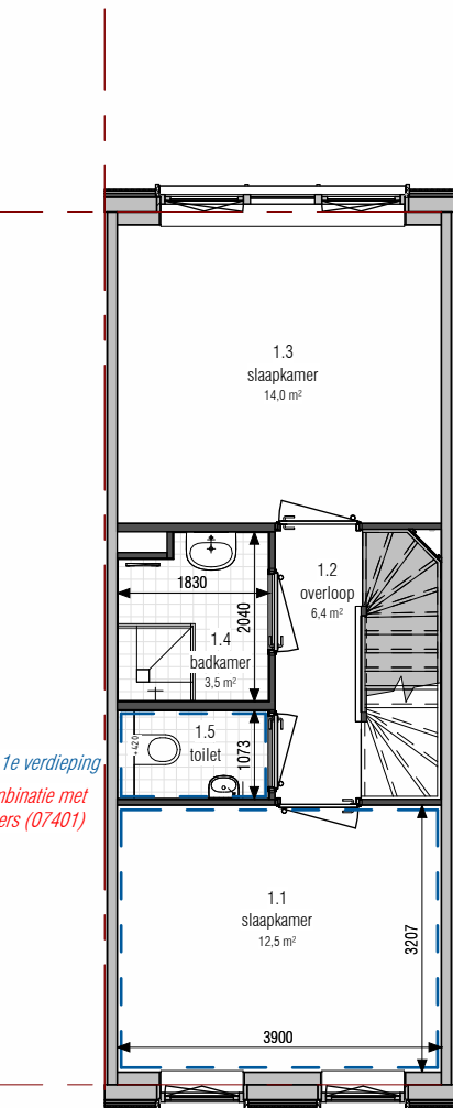
1e verdieping 1 : 100
