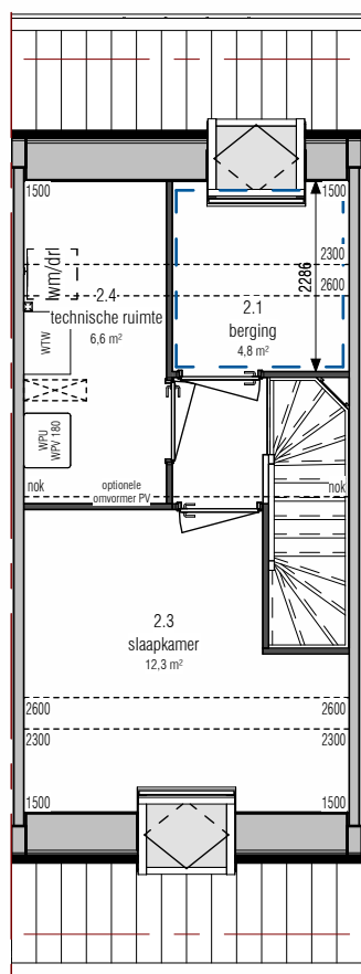
2e verdieping 1 : 100
