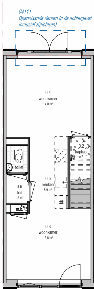
begane grond 1 : 100
