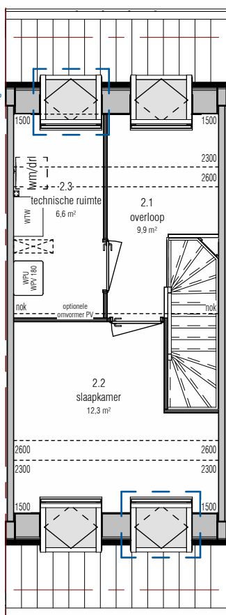
2e verdieping 1 : 100
